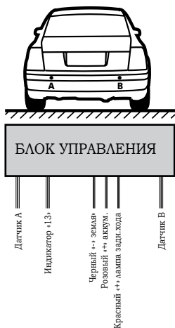
Система с 2-мя датчиками
