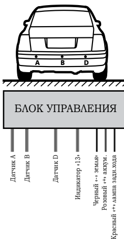
Система с 3-мя датчиками
