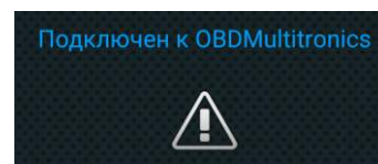
Рис. 3. Успешное подключение
